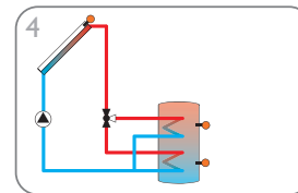
sistema con 1 serbatoio e 1 valvola a 3 vie per il caricamento stratificato del serbatoio (p. 13)
