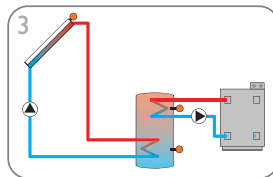
sistema con 1 serbatoio e scambio termico (p. 12)
